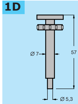
Lampenzieher für T-1 3/4 Lampen. Extractors for T-1 3/4 Lamps.
