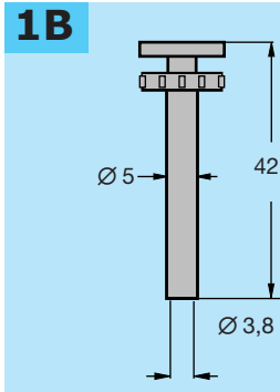
Lampenzieher für T-1 1/4 Lampen. Extractors for T-1 1/4 Lamps.
