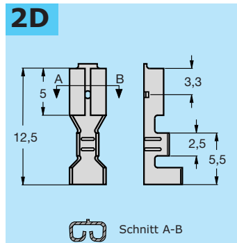
Flachsteckhülse für Steckerbreite 2,8 mm (n. DIN 46330) Receptacle for tab with 2.8 mm (DIN 46330)
